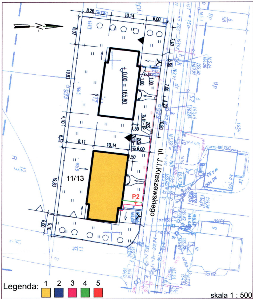
Ryc.7. Strzelin, ul. J.I.Kraszewskiego, dz. nr 11/13 AM-13, wycinek mapy do celów projektowych. Legenda: 1 - usytuowanie budynku mieszkalnego; 2-4 - lokalizacja przyłączy: wodociągowego, energetycznego i kanalizacyjnego; 5 - położenie profilu nr P2.
