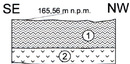
Ryc.5. Strzelin, ul. J.I.Kraszewskiego, dz. nr 11/13 AM-13. Widok na układ nawarstwień zarejestrowanych w profilu nr P1: 1 - szaro-czarna próchnica z gruzem, gliną i żwirem; 2 - żółta glina.
