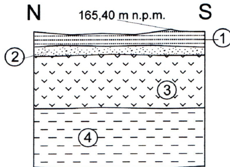
Ryc.6. Strzelin, ul. J.I.Kraszewskiego, dz. nr 11/13 AM-13. Widok na układ nawarstwień zarejestrowanych w profilu nr P2: 1 - szaro-czarna próchnica z gruzem, gliną i żwirem; 2 - szaro-kremowa próchnica; 3 - brązowy żelazo; 4 - żółta glina.
